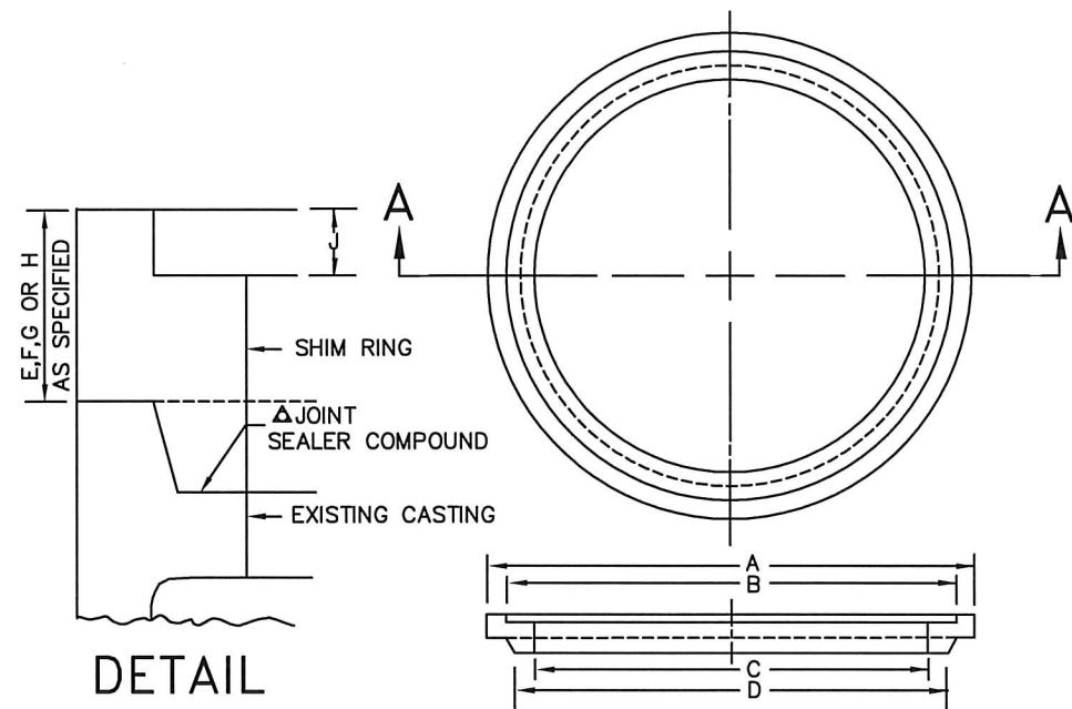
SECTION A-A
